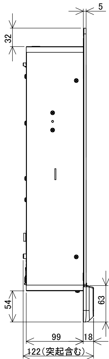
左側面図
