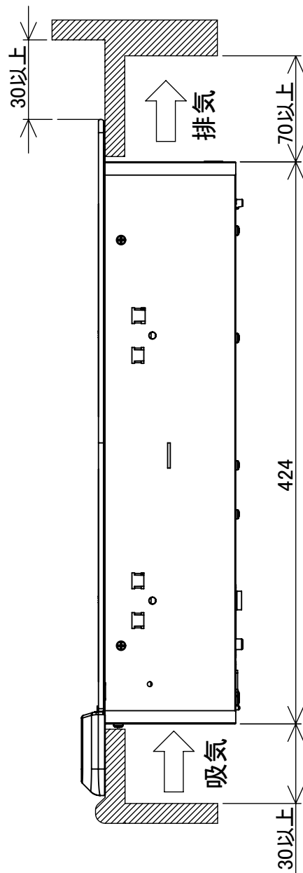
右側面図
