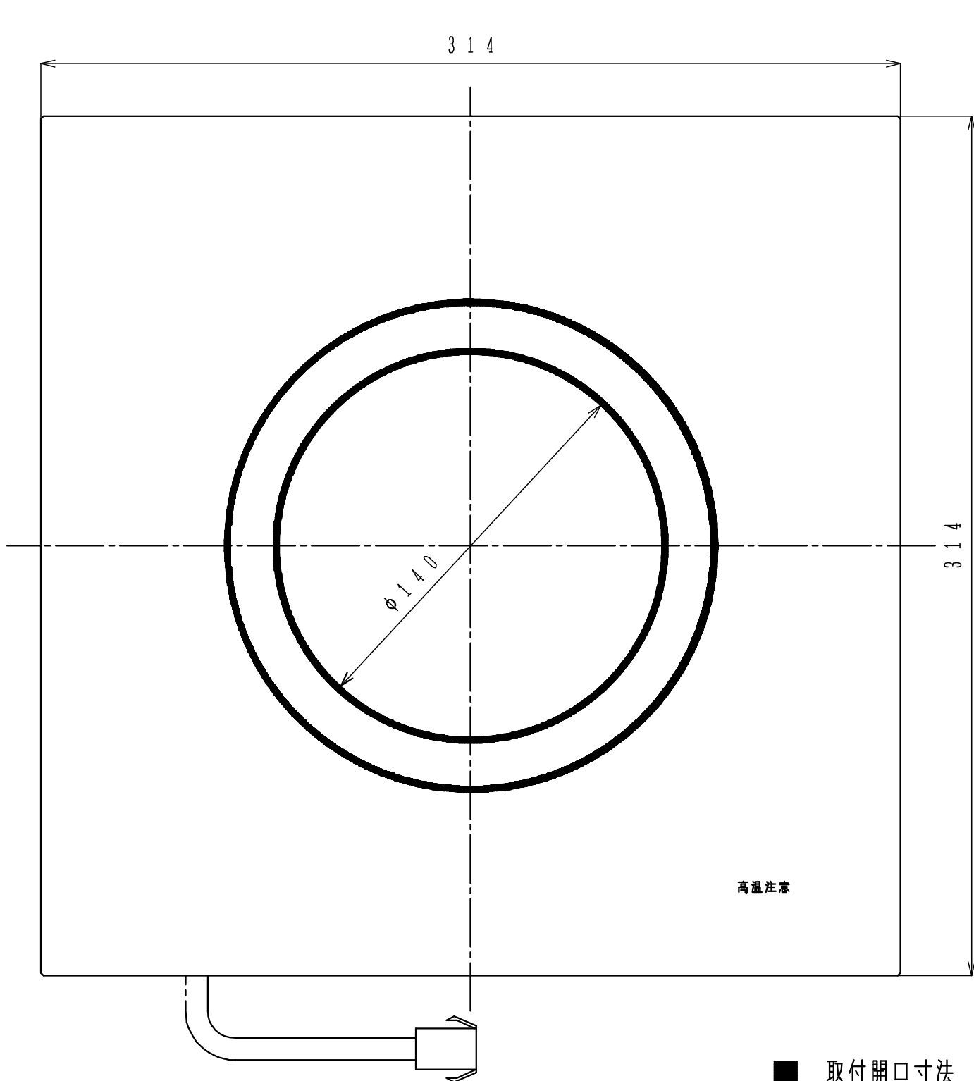
本体
