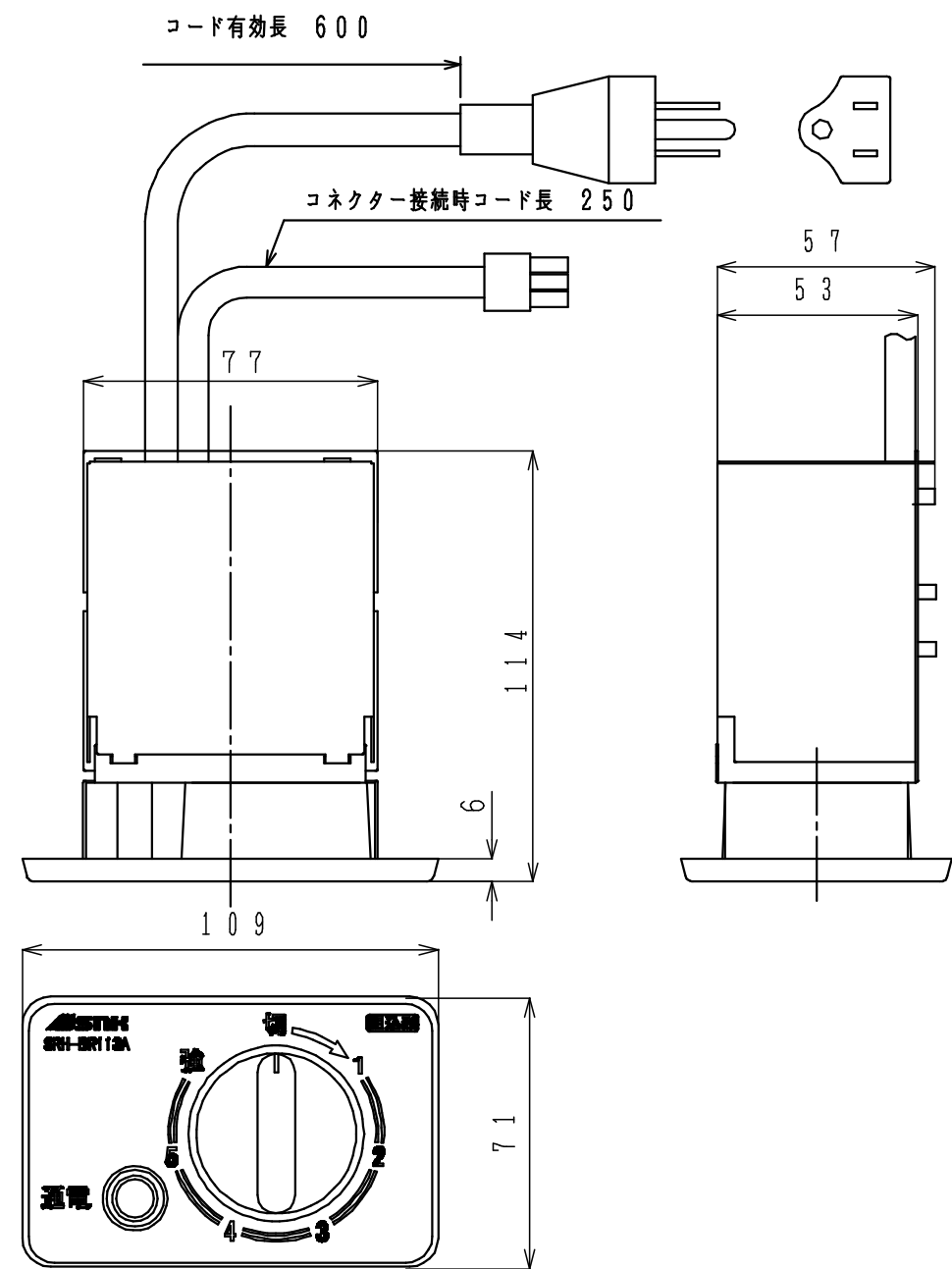
熱量調節器
